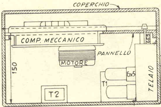
SEZ. LONGITUDINALE
