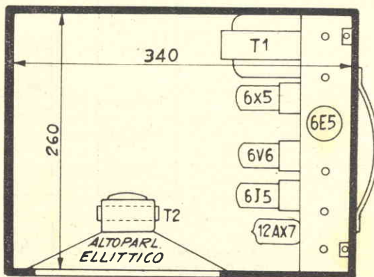
VISTA SUPERIORE SENZA PANNELLO
