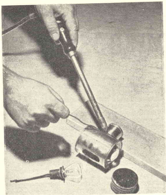
Saldatura del pezzo di tubo destinato ad agire come camino, per creare la corrente di aria di ventilazione. Il foro oblungo, situato in posizione diametralmente opposta a quello per l'aerazione deve essere abbastanza grande per lasciare passare il portalampane.
