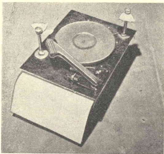
Il cambiadischi completo, prima di essere installato sul mobile.
