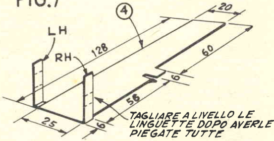
FOGLIA SUPPORTO DISCO PARTICOLARE "B", FARNE 6, TRE CON LINGUETTA A DESTRA, 3 CON LINGUETTA A SINISTRA
