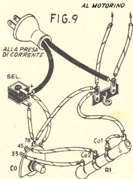
SCHEMA PRATICO DELLA MODIFICA
