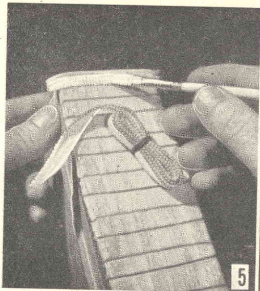
FIGURA 5 - Applicazione dei pezzetti di cimossa colorata, agli spigoli della costola. Essi vanno applicati soltanto dopo che l'intera costola del volume sarà stata coperta abbondantemente di mastice alla para, lasciata seccare e lisciata alla perfezione con cartavetro. FIGURA 6 - Prendere un rettangolo della garza apprettata di dimensioni tali che risulti in totale 25 mm. più corto e 50 mm. più largo della costola. Applicare un altro poco di mastice e premervi sopra la garza. Attendere l'essiccazione, poi togliere per un momento i cartoni, stendere sotto di essi la porzione sovrabbondante della garza e rimmetterli dopo avere applicato pochissimo altro mastice.
